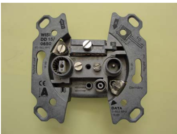
Wisi-Datendose
